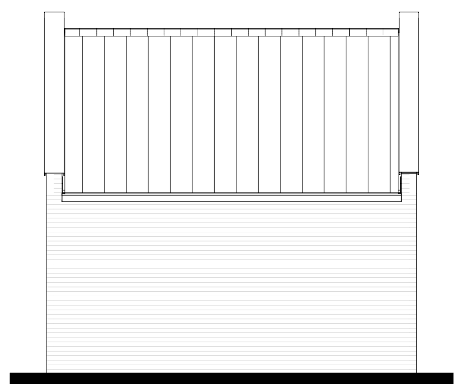
Achtergevel
