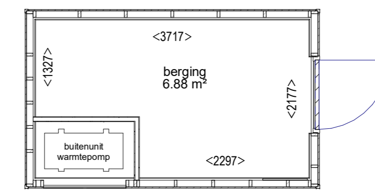
Begane grond
