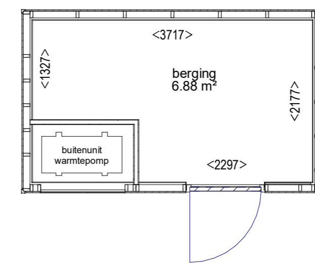
Begane grond
