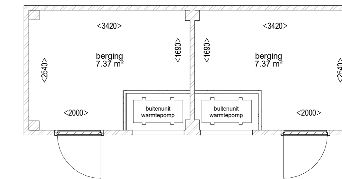
Begane grond
