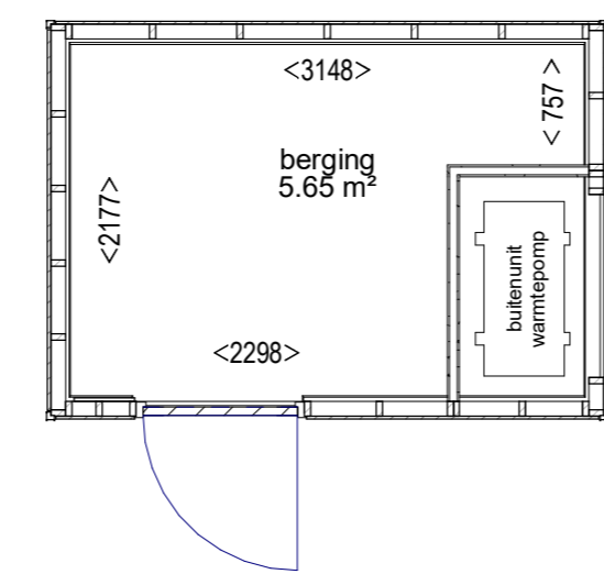
Begane grond
